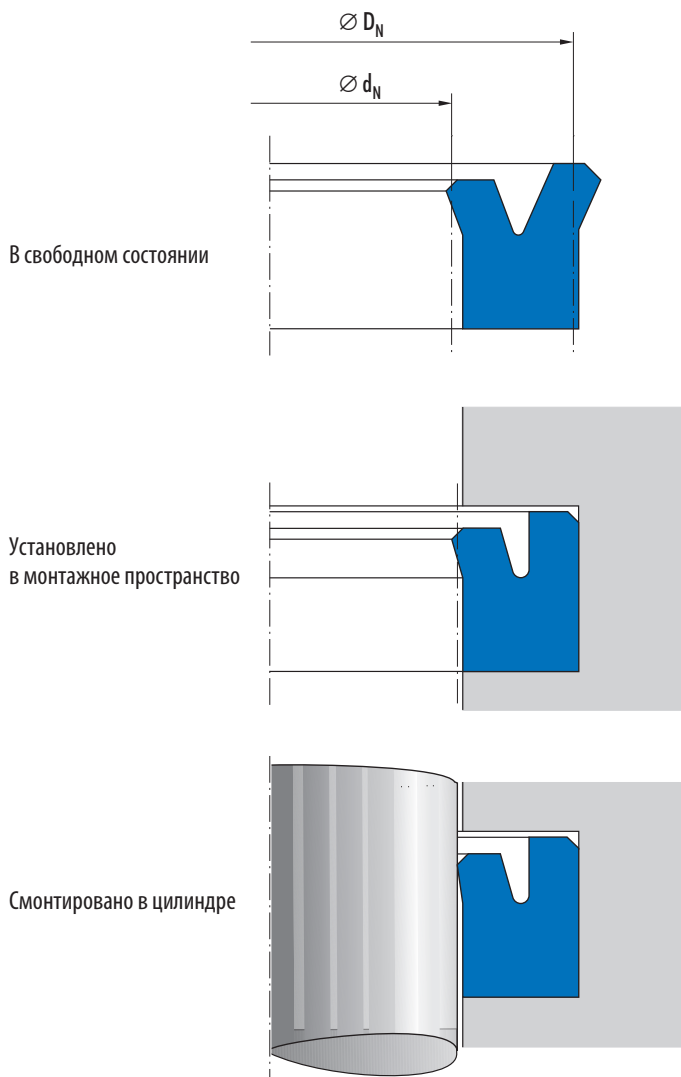
Рис. 4.2 Уплотнение штока
