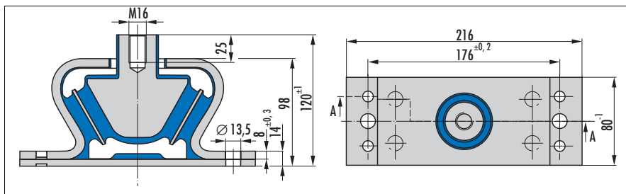
Рис. 18.42 Клиновидная опора 3318 720
