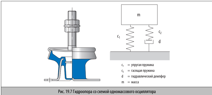
Рис. 19.7 Гидроопора со схемой одномассового осциллятора
