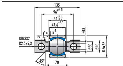
Рис. 18.7 Сферическая опора 5418 710, 711
