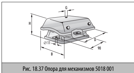
Рис. 18.37 Опора для механизмов 5018 001
