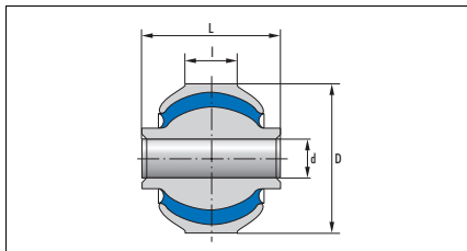
Рис. 18.5 Сферические опоры 5418 036, ...068, ...191, ...070
