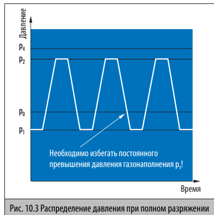
Рис. 10.3 Распределение давления при полном разрядении
