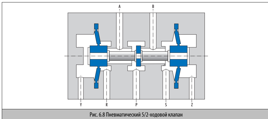
Рис. 6.8 Пневматический 5/2-ходовой клапан
