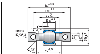
Рис. 18.8 Сферическая опора 5418 732
