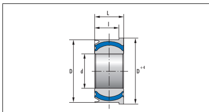
Рис. 18.6 Сферическая опора 5418 163
