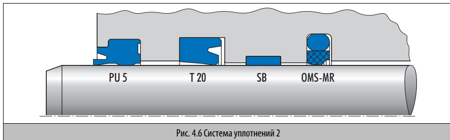
Рис. 4.6 Система уплотнений 2
